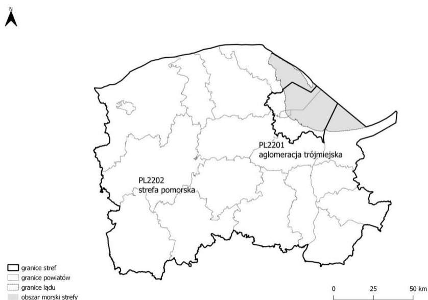
Rys. 5 Podział województwa pomorskiego na strefy dla celów oceny jakości powietrza za 2023r. Źródło: Roczna Ocena jakości powietrza w województwie pomorskim- raport wojewódzki za rok 2023
